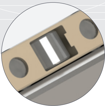
POM (KRE) & PEEK (KREV) KÄFIG FÜR HY (HYBRID) ROLLEN KERAMISCH
